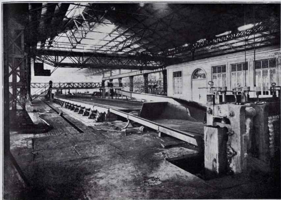
Tren continuo. Uno de los más modernos adelantos que se conocen en la industria siderúrgica. Instalado en la Fábrica de Sestao de la Sociedad Altos Hornos de Vizcaya.
