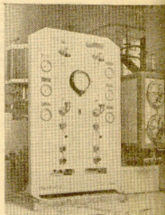
instalación de frío para la mejora y estabilización del vino por un primer tratamiento realizado en proceso de envasado
