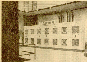
Cuadro de controlización y distribución. Permite el trabajo entre todos los depósitos de la bodega evitando manipulaciones peligrosas para la pureza de los vinos
