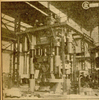
Torneo automático de 2.000 toneladas para forja de bandajes y ruedas.
