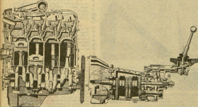
En su gran posición apreciables el grupo motor, a la izquierda del factor, y la caja de cambios. Ambos elementos mecánicos pertenecen al modelo SEAT 132-1.800.
