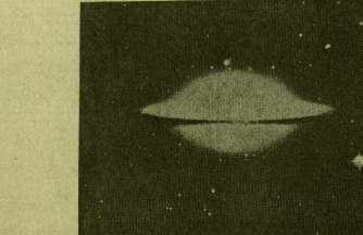
NUESTRA VECINA EN EL UNIVERSO. — A 2 millones de años luz de la galaxia de Andrómeda es la nuestra. Está basada por John Alcock, de polo cúbico. Tiene dos galaxias satélite (arriba y abajo), ligadas a grandes masas de Magellanes. Fotografía tomada con el telescopio Schmidt, de 4 metros, de montas Palomar.
