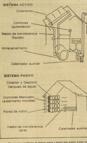
Los esquemas simplificados de sistemas activos y pasivos para producir energía solar
