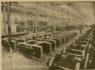
Línea de montaje de bogies para la República Argentina
