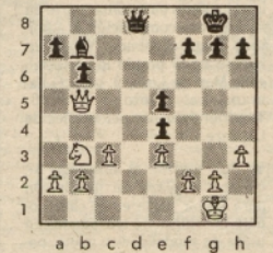
Posición tras 23 Ds5.
