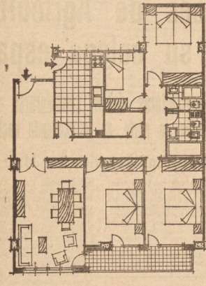
Avenida de Isabel II (avenida de iguales dimensiones que las más amplias del ensanche de Amara). - Tres extraordinarios bloques de viviendas y bajos comerciales. Insertamos el plano de una de las viviendas.
