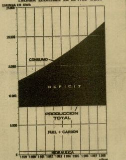
CUADRO N.º 1 Balance Energético del País Vasco a plena utilización de los Medios Propios (En millones de kWh)
